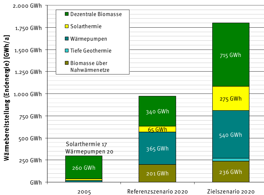
Abbildung 30: Wärmebereitstellung aus dezentralen Erneuerbaren Energien im Referenz- und Zielszenario (gebäude- und nahwärmebezogen) 53
