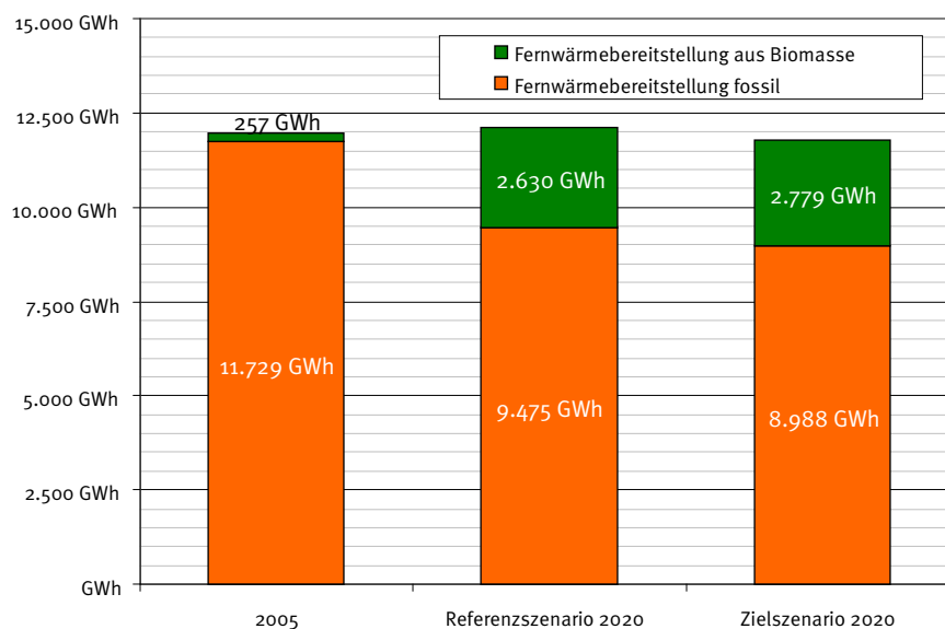
Abbildung 29: Beitrag Erneuerbarer Energien zur Fernwärmeerzeugung im Zielszenario
