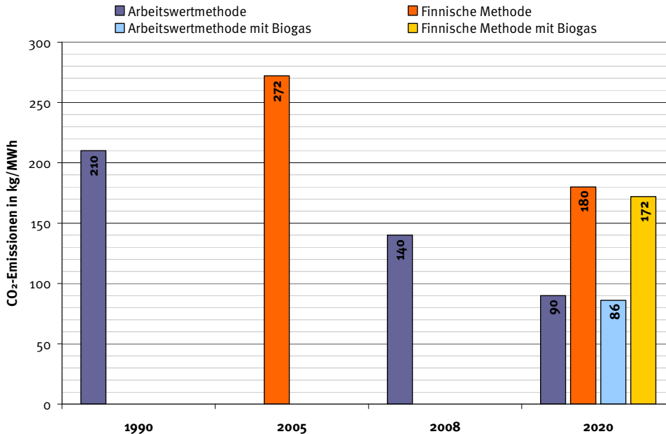
Abbildung 17: CO 2 -Emissionsentwicklung der Fernwärme der Vattenfall Europe AG
