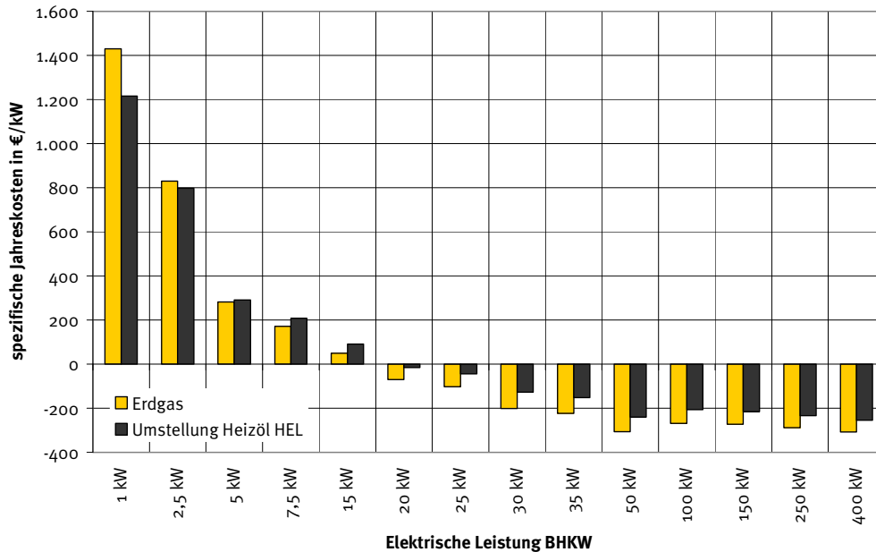
Abbildung 36: Jahreskostendifferenz bei BHKW-Einsatz
